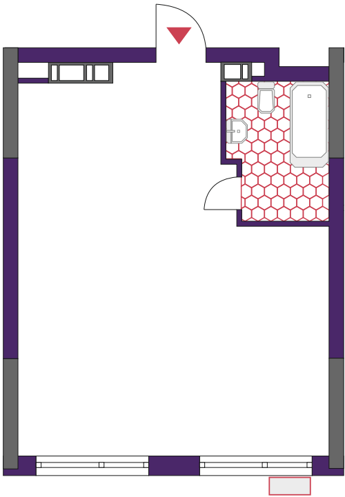
План квартири без перегородок
